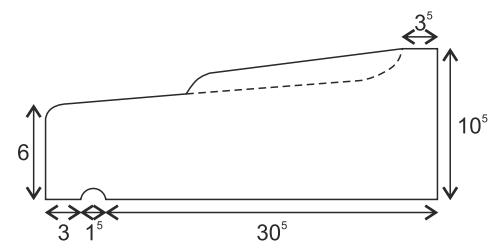
Appui profondeur 35 cm (poids au ml 50 kg)
