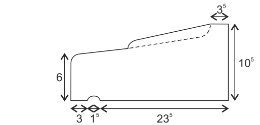
Appui profondeur 28 cm (poids au ml 48 kg)
