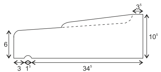
Appui profondeur 39 cm (poids au ml 55 kg)
