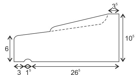
Appui profondeur 31 cm (poids au ml 50 kg)
